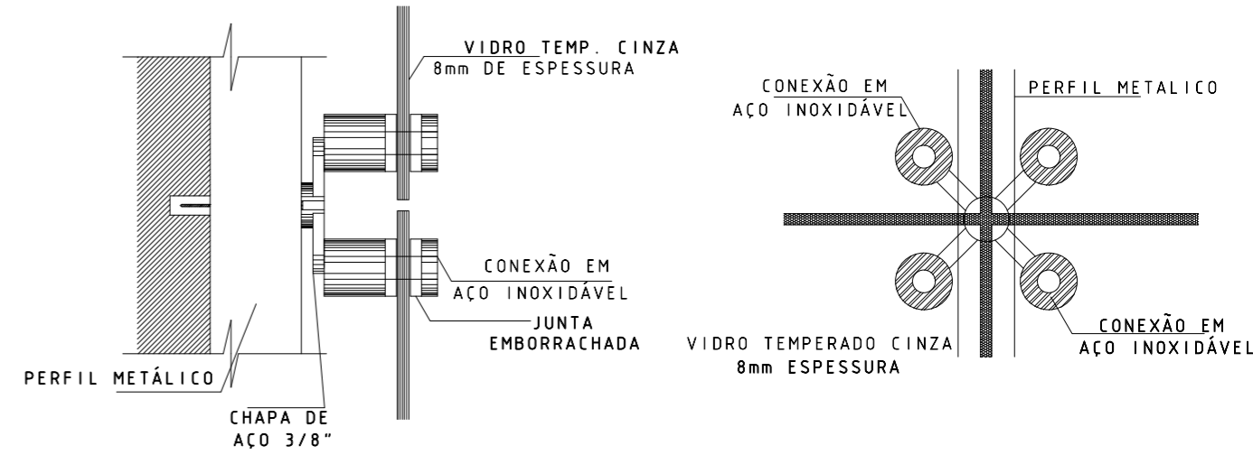
DETALHE 3
