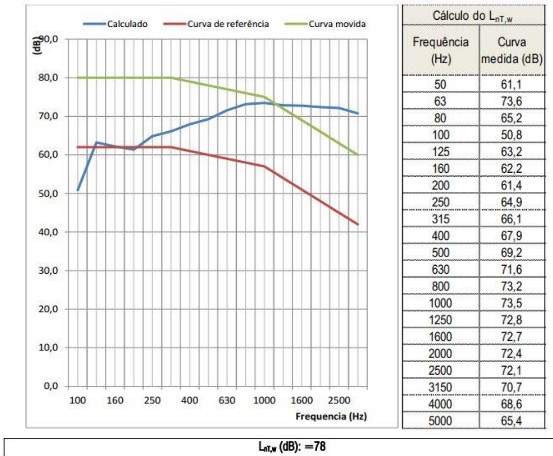
Gráfico 1 - Resultado das variações acústicas internas
