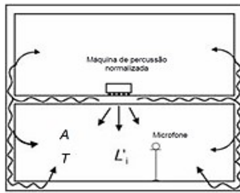
Figura 19 - Esquema de medição
