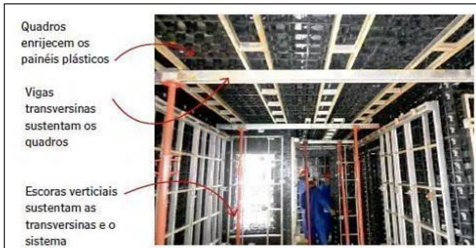
Figura 7 - Fôrmas plásticas
