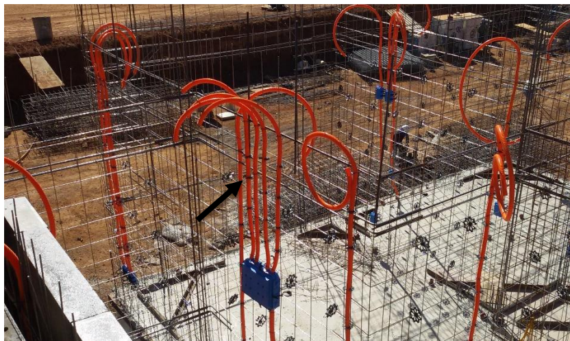
Figura 10 - Espaçadores nos eletrodutos
