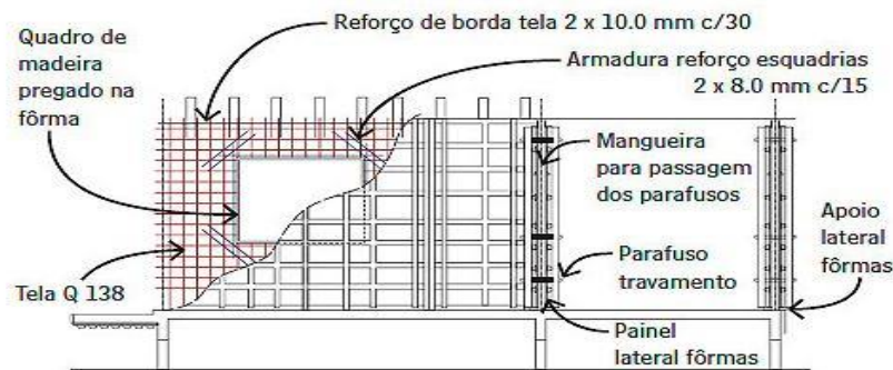
Figura 4 - Vista esquema execução paredes de concreto
